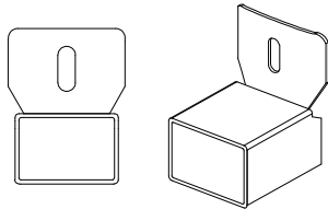
'R' 브라켓 상세도 SCALE : NONE
